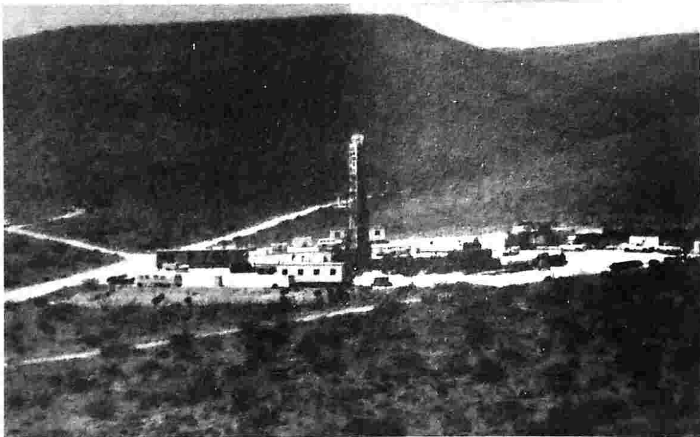
تأسیسات دفع زباله‌های هسته‌ای پیشنهاد شده کوه یاکا در نوادا. این مکان به عنوان مکان بالقوه دفع زباله‌های با پرتوزایی بالای کشور در دست تحقیق است.
