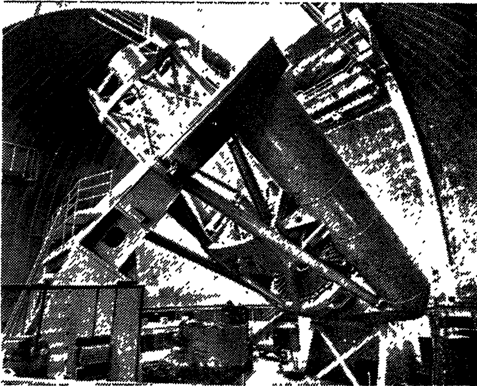
رصدخانه پالومر وابسته بدانشگاه کالیفرنیا
