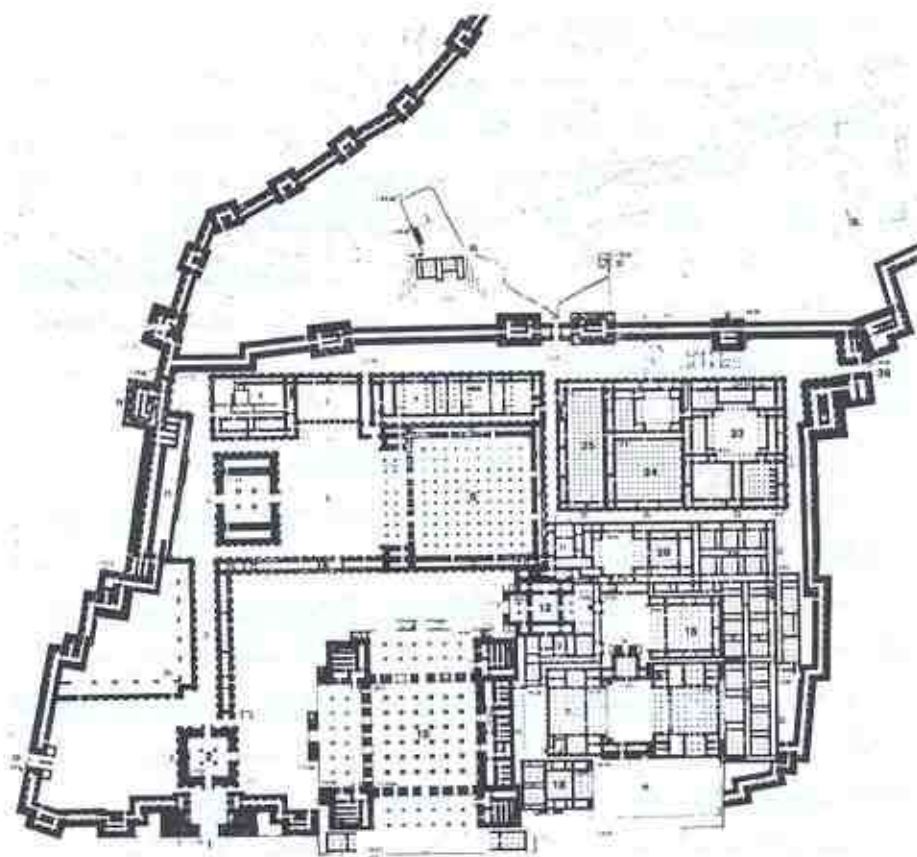
تصویر ۹۲: نقشه‌ی تخت جمشید در زمان هخامنشیان متأخر. بناهای مهم عبارت است از: ۱. پلکان بزرگ غربی؛ ۲. دروازه‌ی ملل؛ ۶. تالار صدستون؛ ۱۰. آپادانا؛ ۱۲. سه دروازه؛ ۱۶. کاخ خشایارشا؛ ۱۸. کاخ داریوش؛ ۲۰. حرم سرای خشایارشا؛ ۲۲. عمارت خزانه، قسمت قدیمی؛ ۲۳. خزانه، با بخش تکمیلی؛ ۲۵. خزانه، با اولین بخش تکمیلی؛ ۲۶. دروازه‌ای در جنوب شرقی، راه نهایی خزانه
