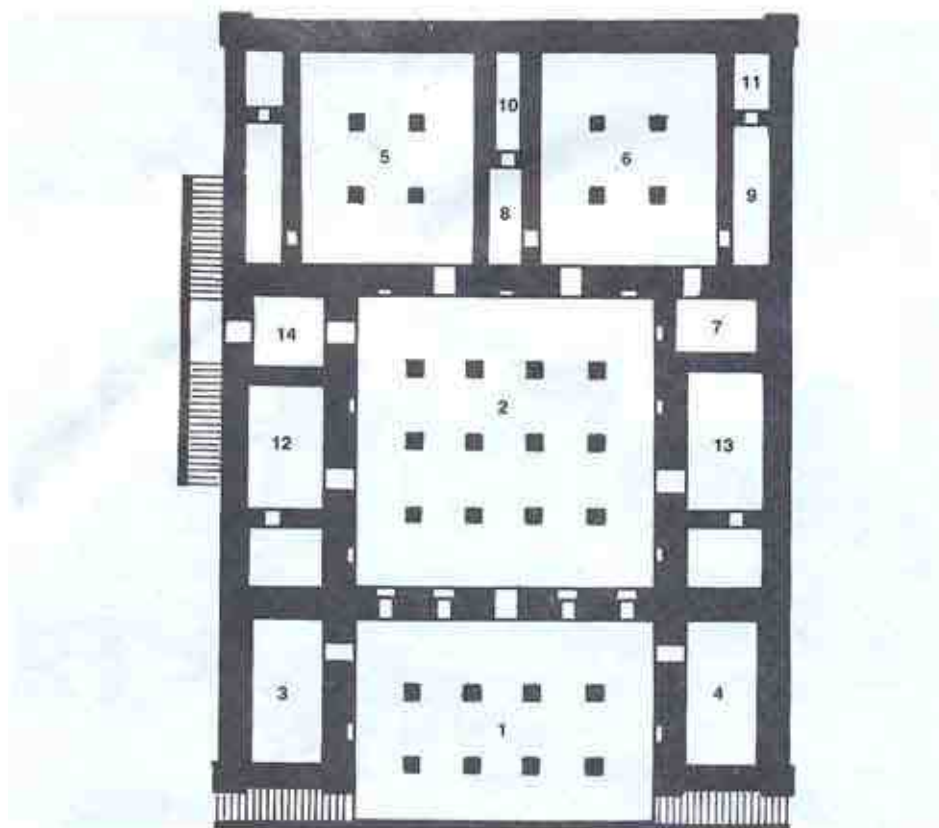
تصویر ۸۶. نقشه ی کاخ داریوش - ۱. ایوان ورودی جنوبی یا دو پلکان - ۲. تالار میانی ۳ و ۴. اتاق نگهبانی ۵ و ۶. اتاق های کنار و استراحت شاه در جبهه ی شمالی ۷ و ۱۱. اتاق های جانبی تالار شماره ی ۱۲ و ۱۳. اتاق های بزرگ کناره ی تالار مرکزی که در برگاه های هر کدام از آن ها پهلوانی در حال نبرد با حیوان افسانه ای تکر شده است ۱۴. در ورودی جانبی در سمت غرب
