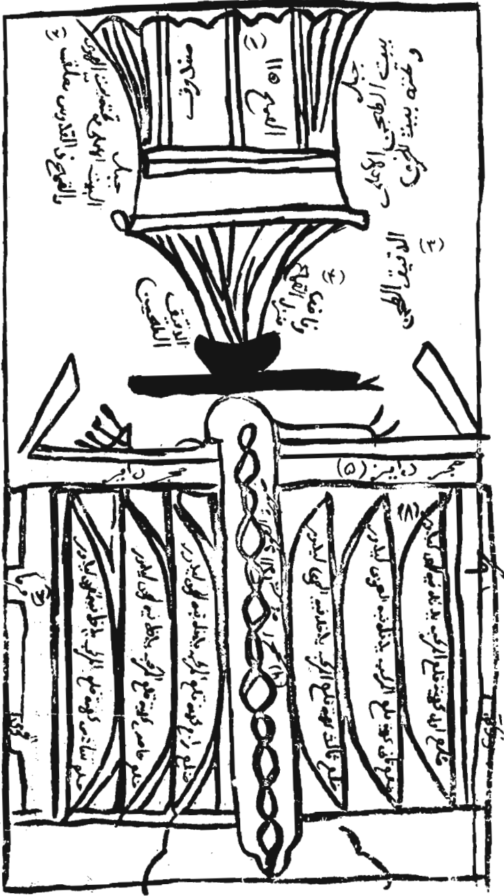
۱. صندوق القمح: صندوق کندم ۲۰. جیل بیت الطحین الاعلی و تحته بین الهوی والقمح فی القادوس معلق. قسمت بالای اطاقک زبرین آسیاب که اطاقک هوا زبران قرار دارد و کندم در میان سید یا صندوقی ریخته و آویخته می گردد. ۳. الدقیق الطحین: آرد ۴۰. فاض منزل القمح. پوستی قیف مانند که کندمها را روی سنگ زبرین آسیاب می ریزد. ۵. حجر دایر: سنگ زبرین آسیاب که می گردد. ۶. صوره العمود الدایر به الحجر: نمای دیرکی که سنگ آسیاب به وسیله آن می چرخد. ۷. مرما (مرمی، همچنانکه در متن آمده) الهوی: روزنه هوا و هواکش ۸. ضلع اول ۱۰۰. کهبیشه قلع المركب یدخل فیهِ الهوی لیدور: پره یکم تا ششم که همانند بادبان کشتی هستند و باد در آنها داخل می شود تا به چرخش درآیند.
